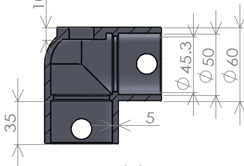
断面図 A-A スケール 1 : 3
