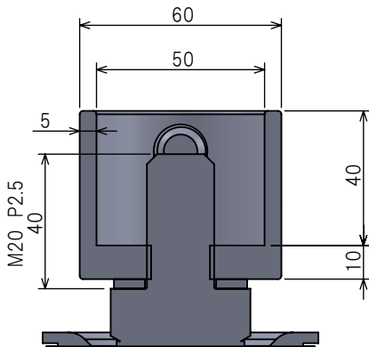
挿入部断面 スケール1:2
