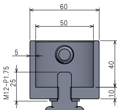
挿入部断面 スケール1:2
