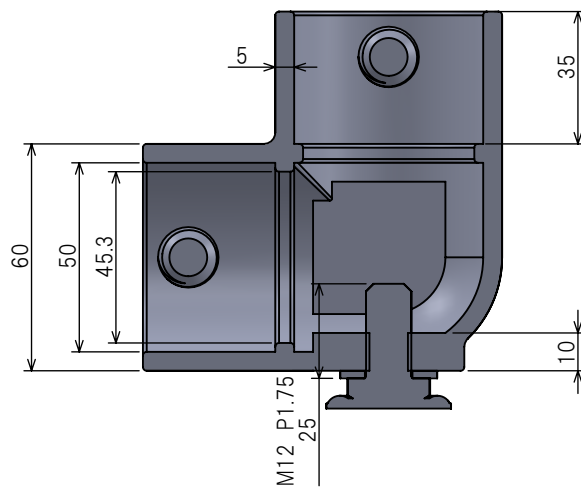
挿入部断面 スケール1:2
