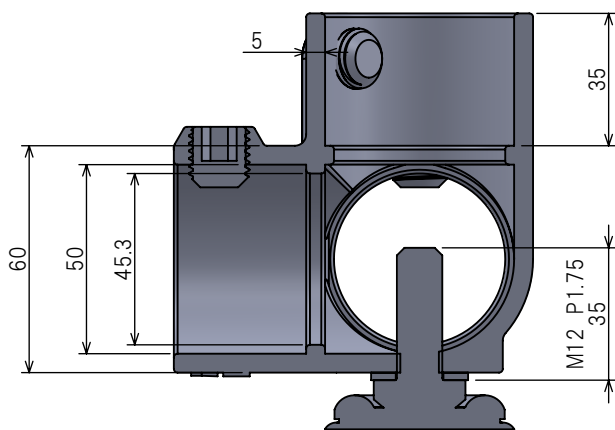
挿入部断面 スケール1:2
