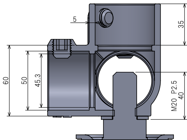
挿入部断面 スケール1:2
