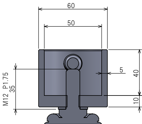
挿入部断面 スケール1:2
