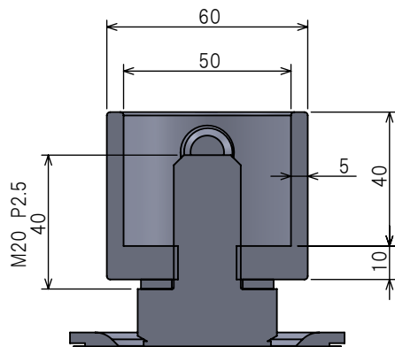
挿入部断面 スケール1:2
