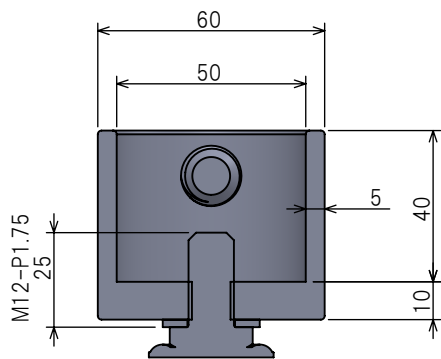
挿入部断面 スケール1:2
