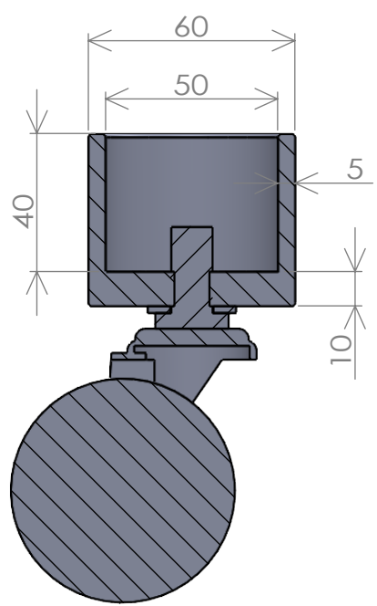
断面図 A-A
