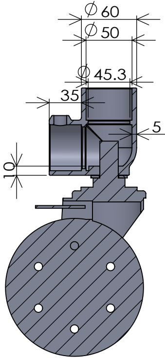
断面図 A-A スケール 1 : 4
