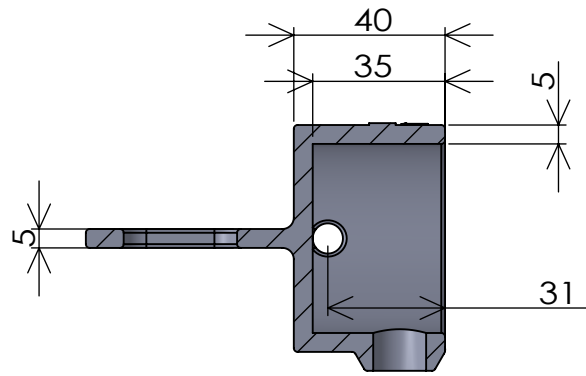
断面図 R-R
