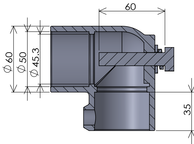
断面図 R-R
