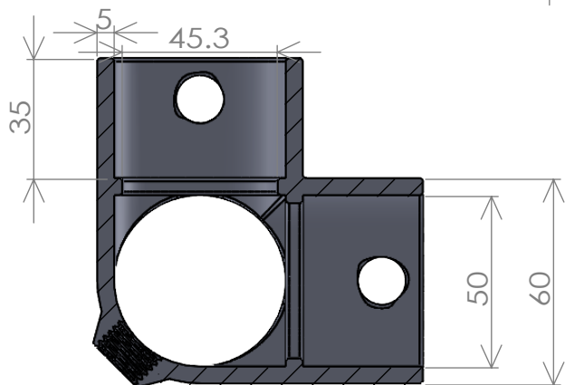
断面図 A-A
