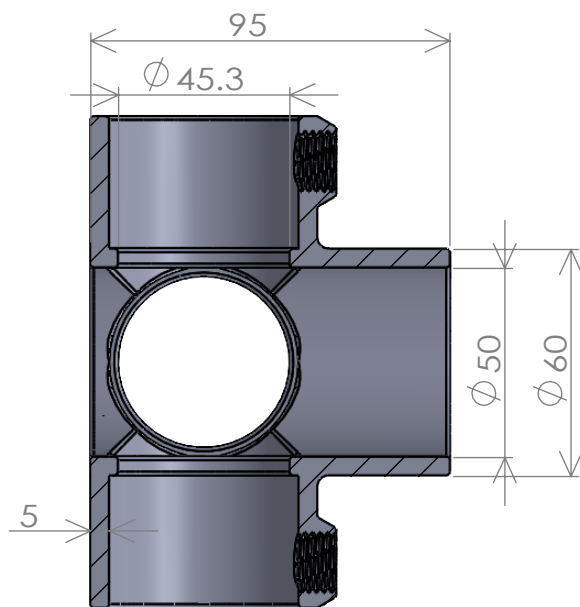
断面図 A-A
