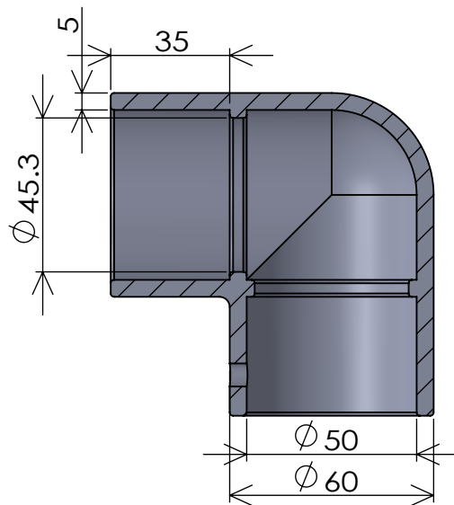
断面図 R-R
