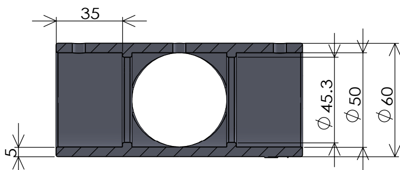
断面図 R-R
