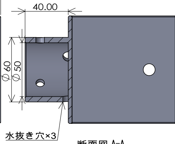
断面図 A-A スケール 1 : 2
