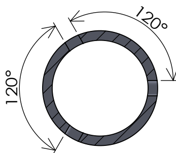
断面図 B-B スケール 1 : 2
