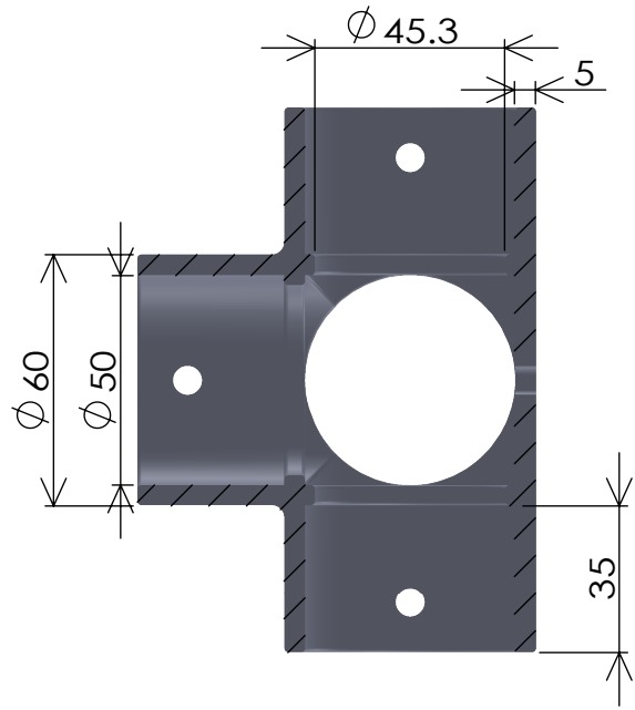
断面図 R-R
