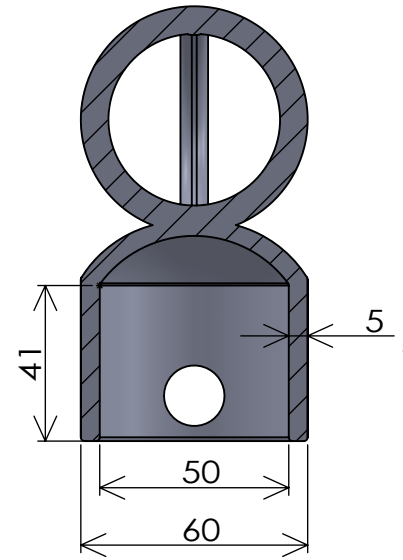
断面図 A-A
