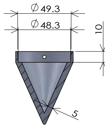
断面図 A-A スケール 1 : 2
